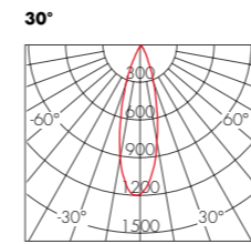
DDO065B 4W
